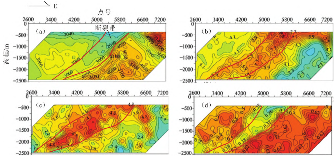
图6 胶东纱岭矿区320勘查线SIP剖面图
