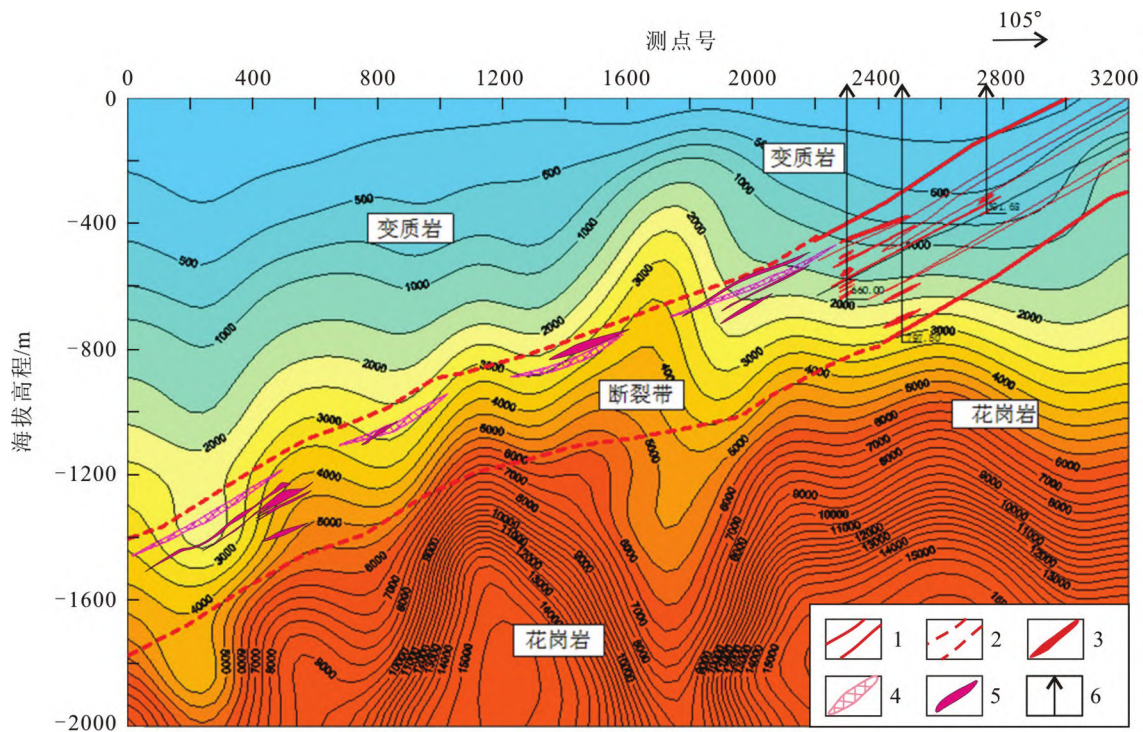
图5 胶东寺庄矿区360线CSAMT法推断解释地质剖面
