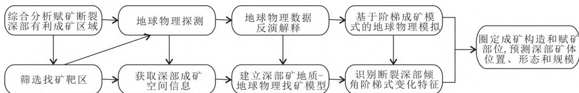
图1 深部阶梯找矿方法流程图
