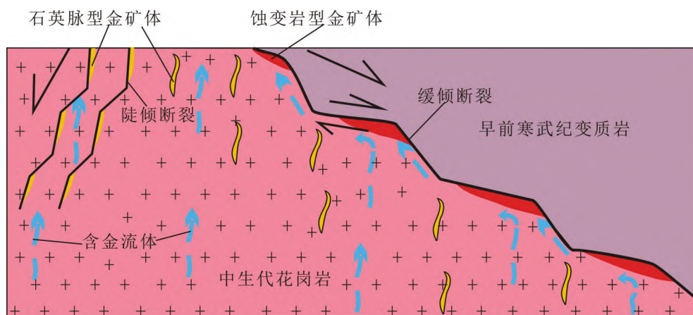
图2 深部金矿的阶梯成矿模式(据宋明春等,2020)
