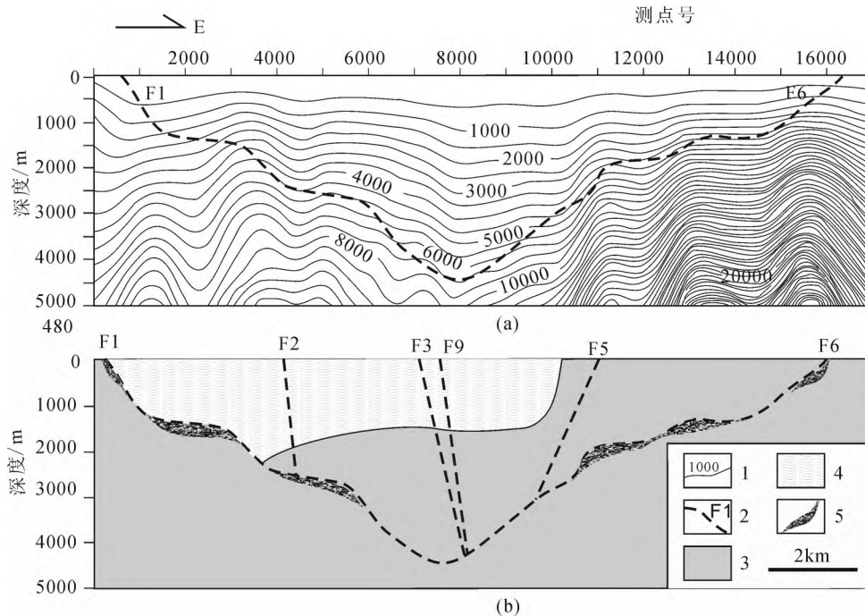
图7 胶东三山岛断裂—焦家断裂大地电磁测深剖面(a)及推断解释地质剖面(b)(据 Song Mingchun et al., 2021)
