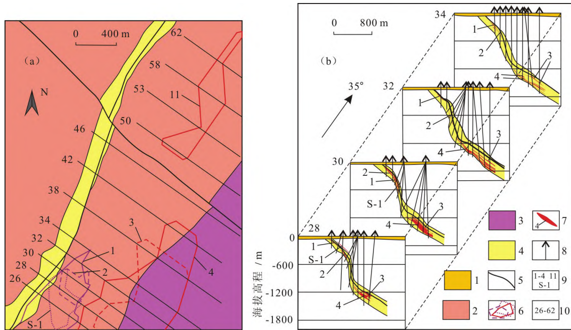
图3 胶东三山岛北部海域超大型金矿床基岩地质图(a)及勘探线联合剖面图(b)(据宋明春等,2015) 1—第四系;2—玲珑型花岗岩;3—新太古代变质岩系;4—破碎蚀变带;5—断裂;6—主要矿体水平投影范围;7—金矿体;8—钻孔位置;9—矿体编号;10—勘探线编号
