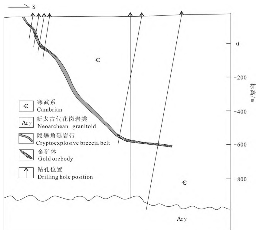
图4 鲁西归来庄金矿床28号勘查线剖面图(据张国权,2017)
