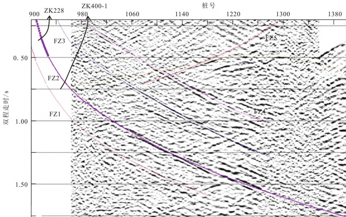
图8 胶东尹家西北矿区反射地震剖面
