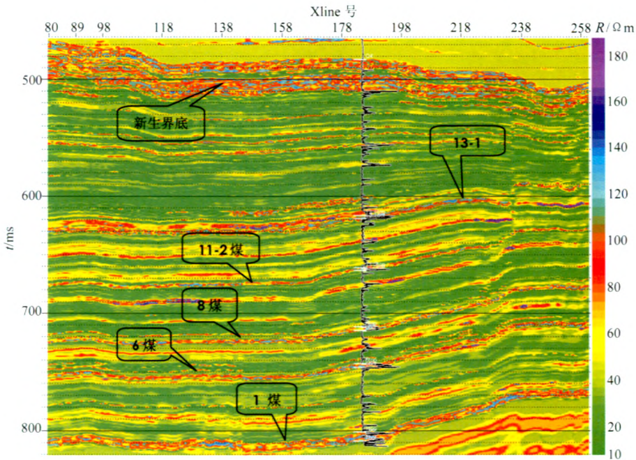
图 4 过补 2 井 113 线电阻率剖面
