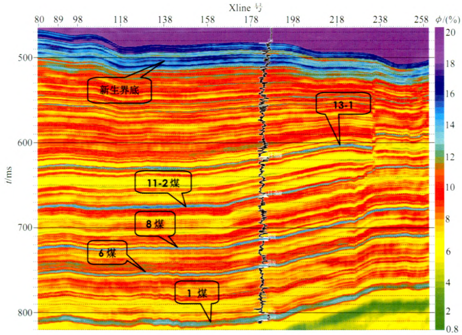
图 3 过补 2 井 113 线孔隙度剖面
