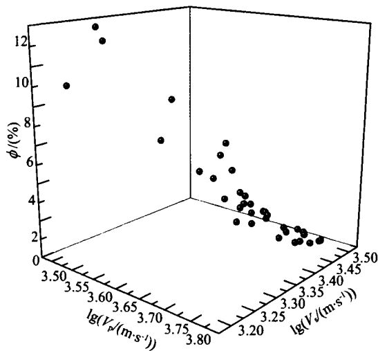
图 1 孔隙度 \phi 与 v_p 、 v_s 的关系(实验数据)
