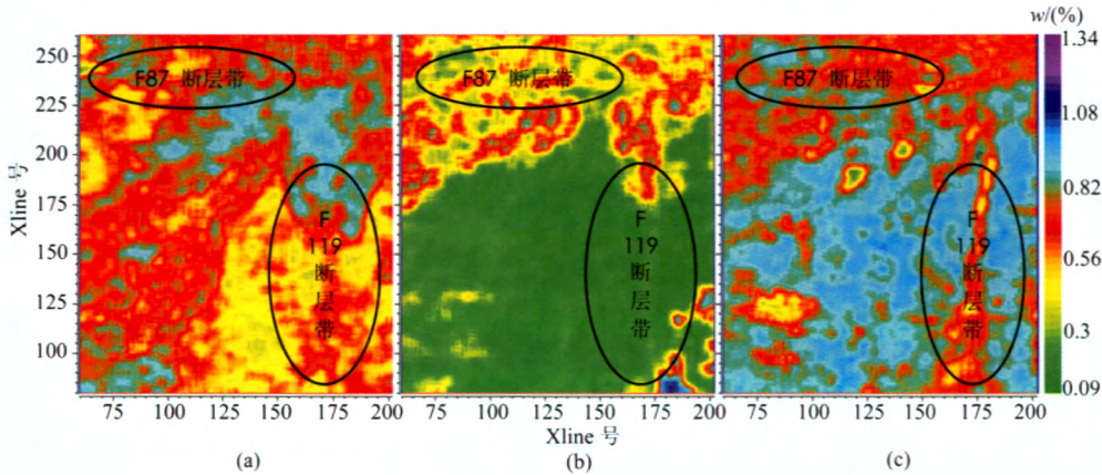
图8 13-1煤及其顶、底板含水量图
