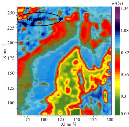
图7 第四系底含水量图
