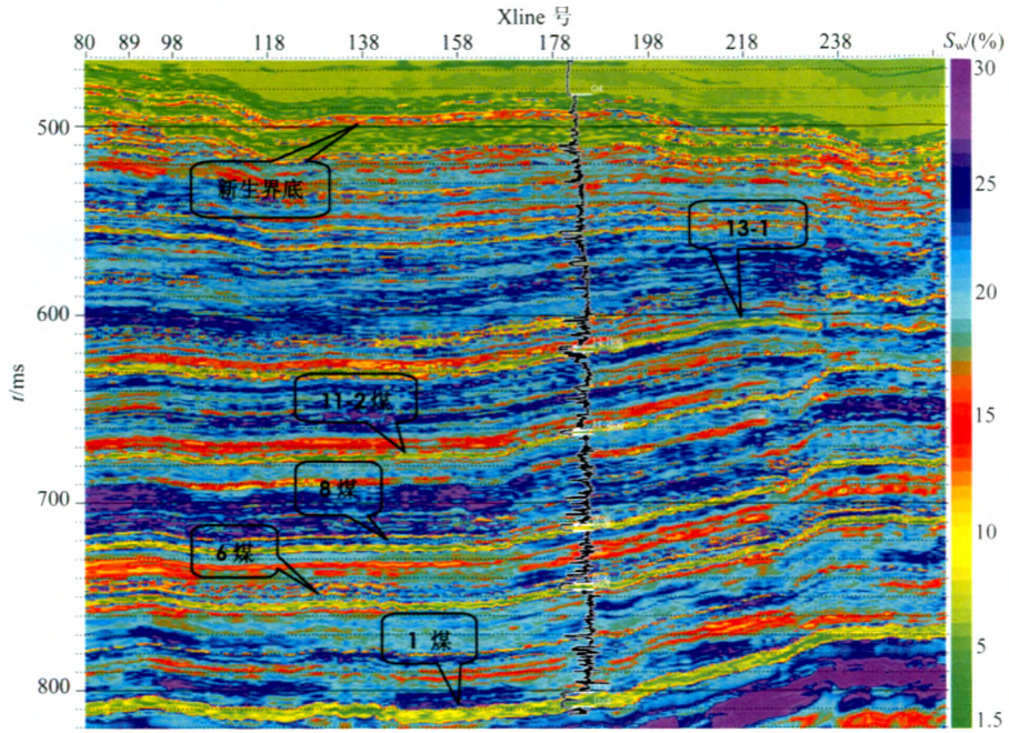
图 5 过补 2 井 113 线相对含水饱和度剖面
