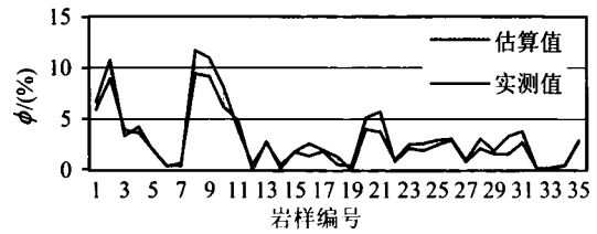
图 2 双波速法求取的孔隙度与实测孔隙度对比
