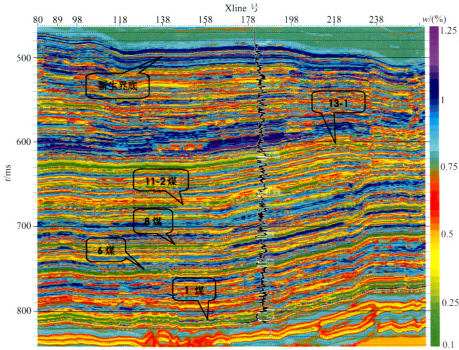
图 6 过补 2 井 113 线含水量剖面
