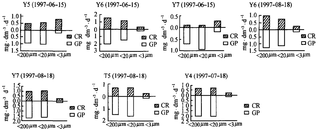
图1 各实验围隔不同粒级浮游生物的呼吸率(CR)及浮游植物的生产率(GP)
