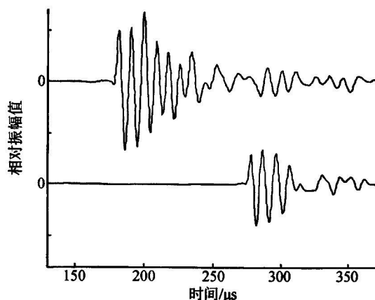
图 4 原位测量系统海水校正得到的信号
