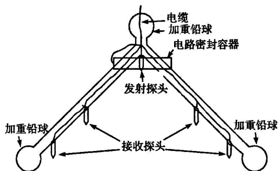
图3 海底部分仪器构造 Fig. 3 Structure of the underwater part
