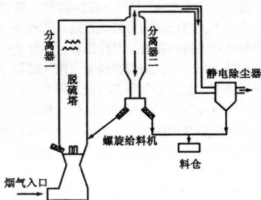
图 1 双循环流化床烟气脱硫工艺流程
