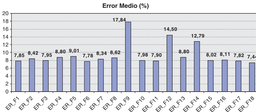
Figura 3 Error medio de la fórmula propuesta y comparación con las fórmulas ya existentes.
