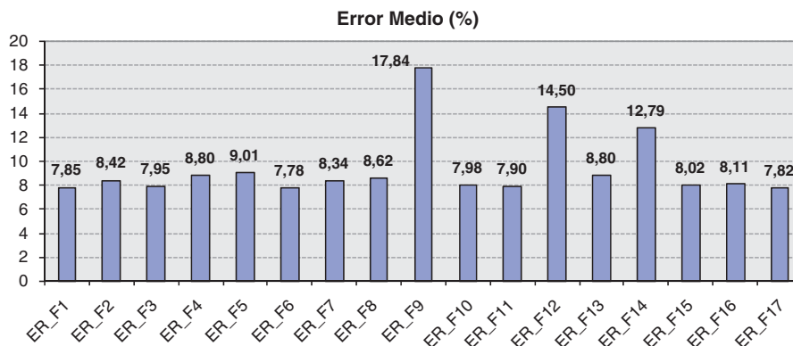
Figura 1 Error medio de las fórmulas analizadas.
