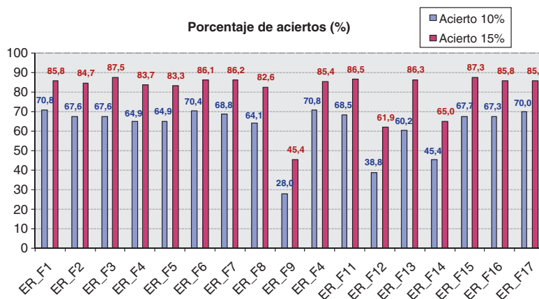
Figura 2 Porcentaje de estimaciones válidas.
