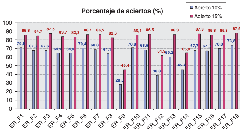
Figura 4 Porcentaje de estimaciones válidas de la fórmula propuesta y comparación con las fórmulas ya existentes.
