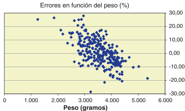
Figura 5 Errores cometidos en función del peso.
